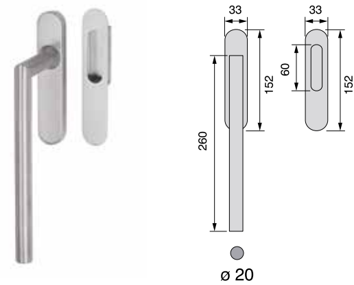
GL-1401IP, üveghez
